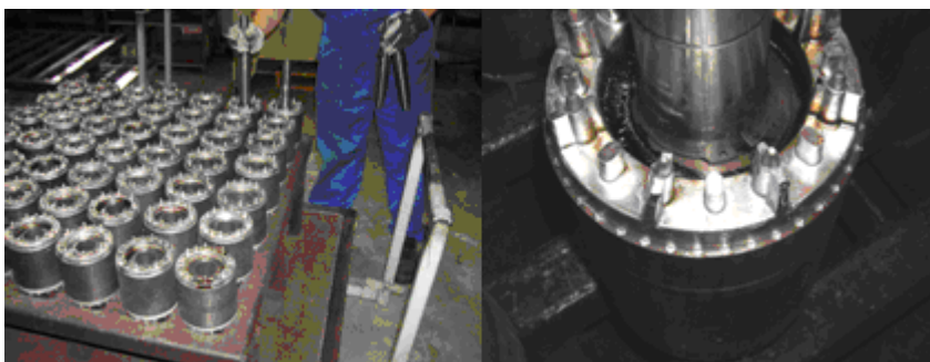
Kuva 1. Vasemmalla roottoripakka lämmitettyä, oikealla akseli liitettyä pakkaan.
